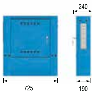
Armadio per allacciamenti
