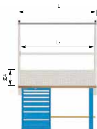
Lunghezza 1250 / 1500 / 1750 mm
