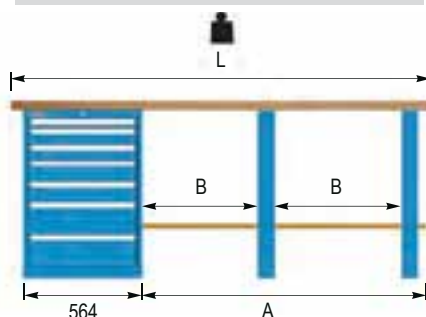
2 Gambe di appoggio e 1 Armadio a cassetti 27x36 Eh
