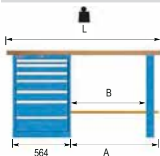
1 Gamba di appoggio e 1 Armadio a cassetti 27x36 Eh
